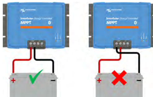
Esempi di polarità corretta ed erranea (inversa) della batteria.
